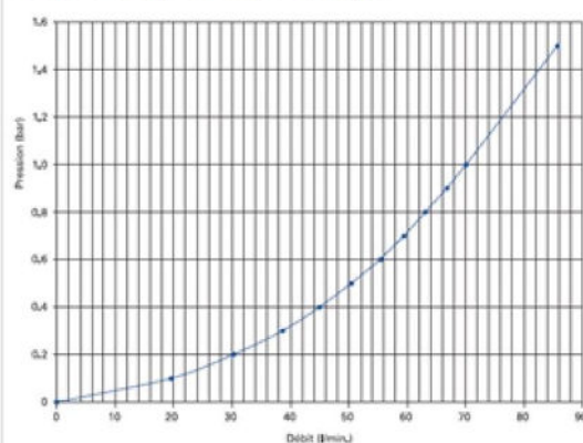
Courbe de pertes de charges
